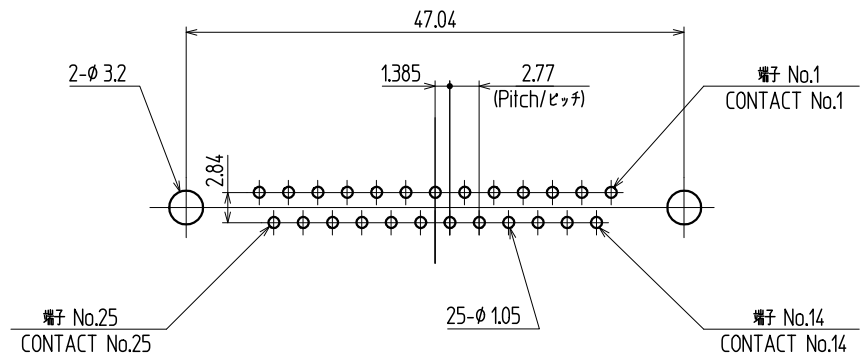
Dimensions of PC board holes / 参考基板孔寸法図 (Printed-side view, Tolerance all ±0.1) / (パターン側より見る 公差±0.1)
