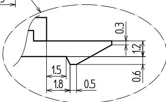
Detail of snap スナップ部詳細図
