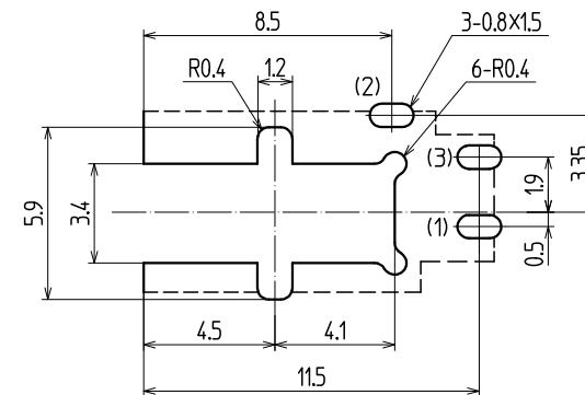
Dimensions of PC board holes / 参考基板孔寸法図 (Parts-side view Tolerance all ±0.05) / (部品側より見る 公差±0.05)
