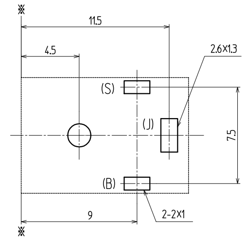
Dimensions of PC board holes / 参考基板孔 Parts side view / 部品面より見る
