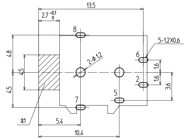
参考基板孔図(部品面) (公差 ALL±0.1)
