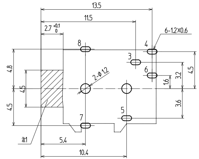
参考基板孔図(部品面) (公差 ALL \pm 0.1 )
