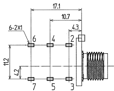
参考基板孔図(部品面) (公差 ALL±0.1)
