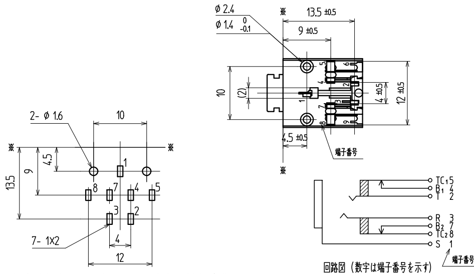
11.6 参考基板孔寸法図 (パターン面より) (公差ALL±0.1) 数字は端子番号を示す
