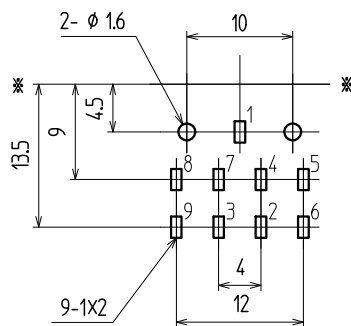
1.6参考基孔寸法図 (パターン面より)(公差ALL±0.1)
