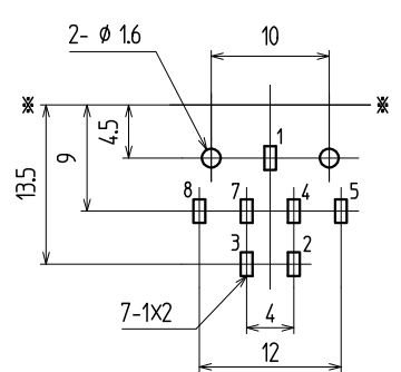
寸法公差 X 6未満 ±0.3 X 6以上 20未満 ±0.4 X 20以上 未満 ±0.5 X 以上 ± 角 度 ± ° 記号 改 訂 事 項 年月日 担当 図1.6 参考基板孔寸法図 (パターン面より) (公差ALL±0.1) 数字は端子番号を示す。
