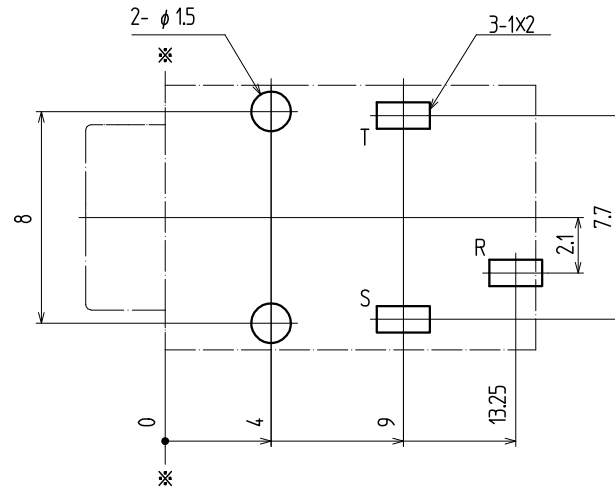
t1.6 参考基板孔寸法図 (パターン面より) 公差 ALL±0.1
