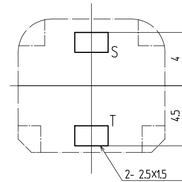
†1.6 参考基板孔寸法図 (パターン面より) (公差ALL±0.1)
