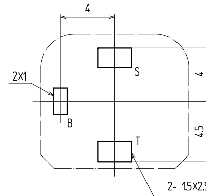
f1.6 参考基板孔寸法図 (パターン側)(公差 ALL±0.1)
