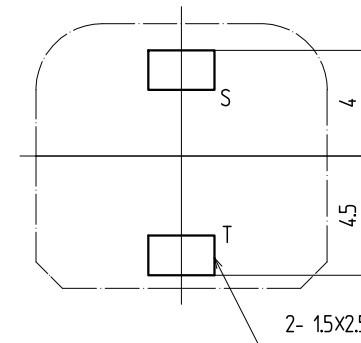
†1.6 参考基板孔寸法図 (パターン側)(公差 ALL±0.1)
