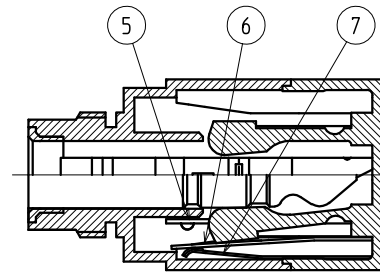
B-B 断面図
