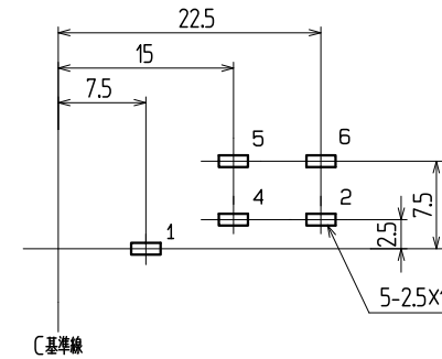
1.6参考基板孔寸法図 (パターン面より)(公差ALL±0.1)
