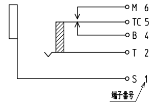
回路図 (数字は端子番号を示す)
