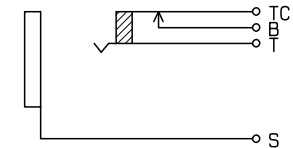
回路図 (数字は端子番号を示す)
