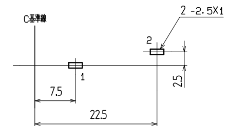
†1.6 参考基板取付寸法 (パターン面)
