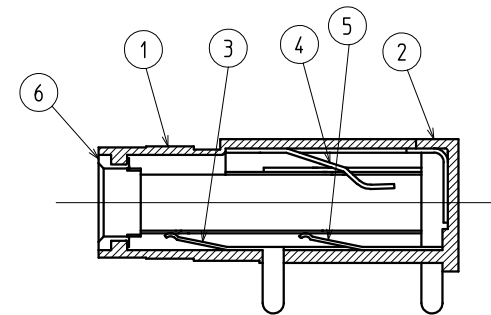
A-A 断面図
