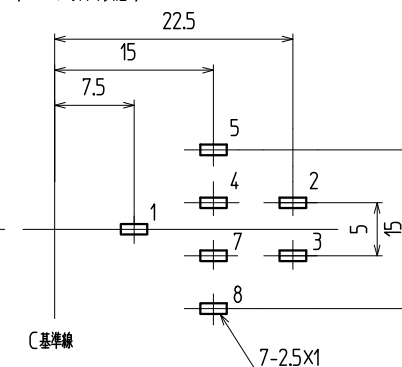
1.6 参考基板孔寸法 (パターン面) (公差ALL±0.1) (数字は端子番号を示す)
