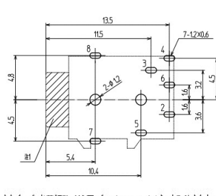
†1.6 参考基板寸法図 (パターン面より) (公差ALL±0.1)
