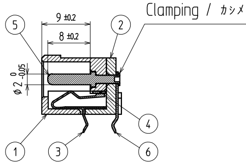
A-A Sec / 断面図
