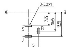
Dimensions of PC board holes / 参考基板孔 Tolerance / 公差 ALL±0.05 Soldering-side view / 半田面側より見る
